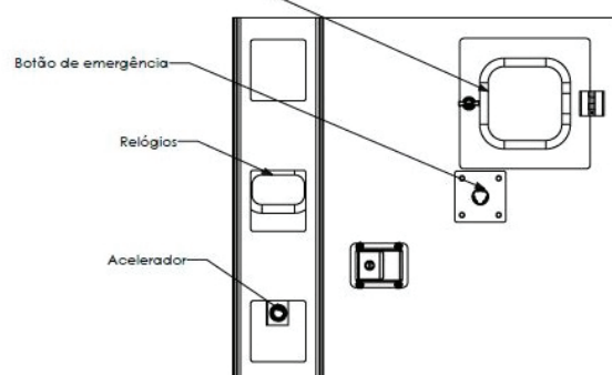
DETALHE F
